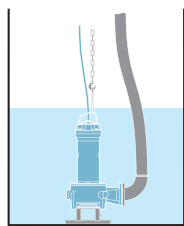
自由式安装
